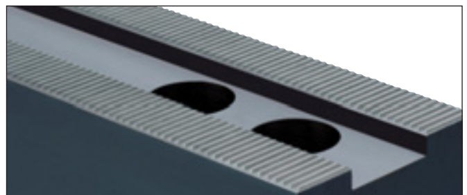
Spannbacken nach der Reinigung / Serrations after cleaning
