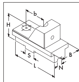
Trägerbacke TRQK...-2 Support Jaw TRQK...-2
