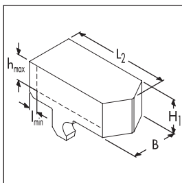
Wechselbacke BWB Soft insert BWB
